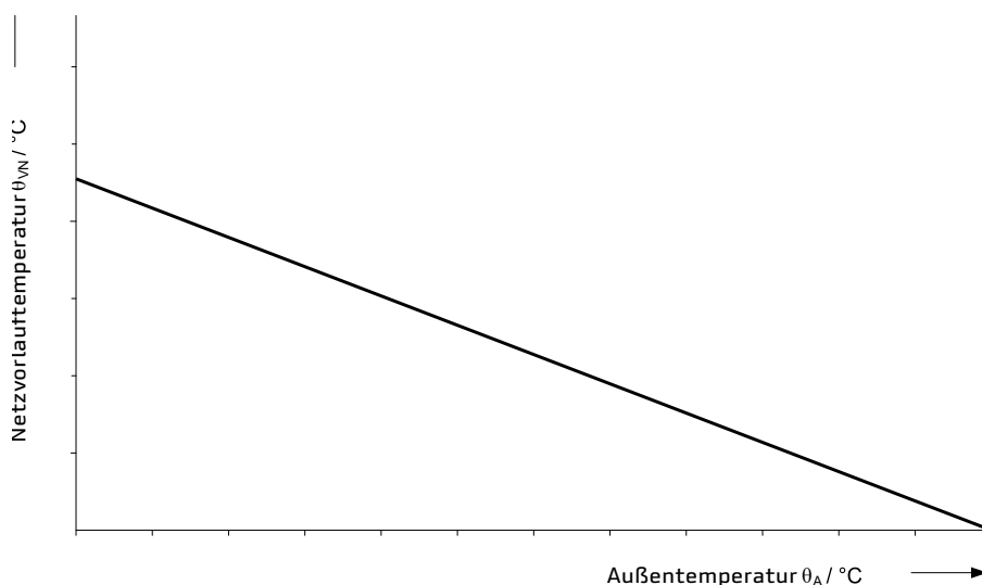
Abbildung 2: Netzzvorlauftemperatur \theta_{vN} in Abhängigkeit von der Außentemperatur \theta_A ; prinzipieller Verlauf einer gleitenden Fahrweise
