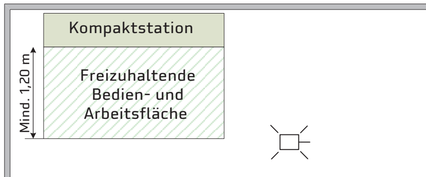
Abbildung 5: Platzbedarf
