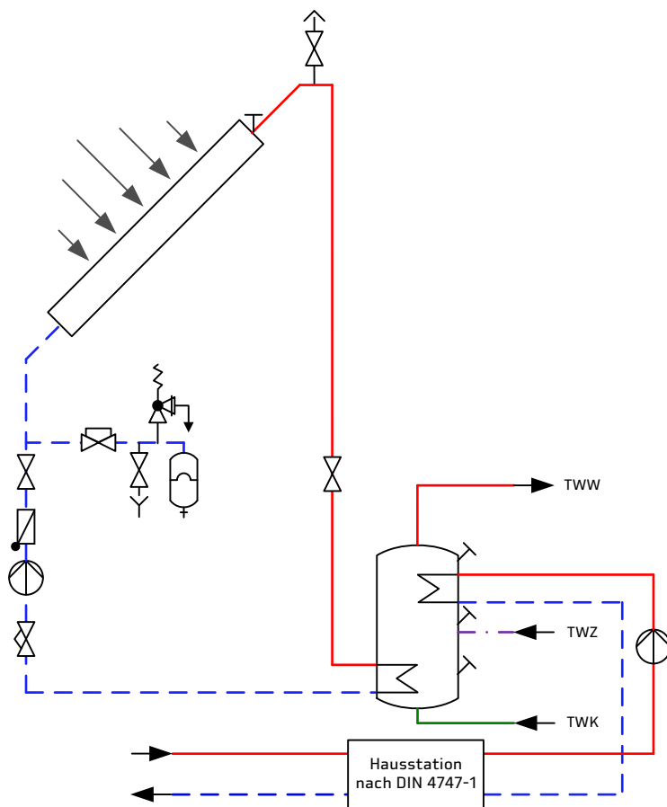
Abbildung 26: Speichersystem mit innenliegenden Heizflächen für Solar und Fernwärme
