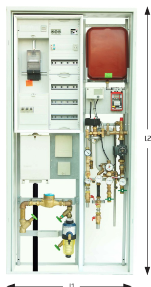
Abbildung 6: Darstellung einer Hausanschlussnische
