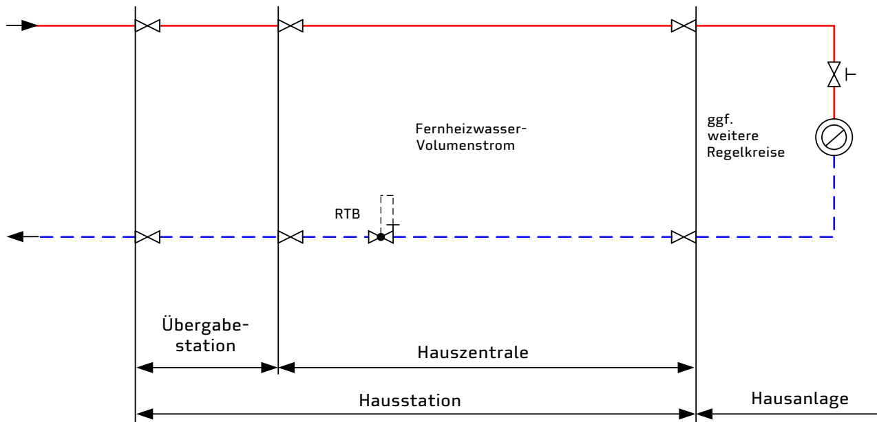
Abbildung 9: Hauszentrale Raumheizung Prinzipschaltbild für den indirekten Anschluss
