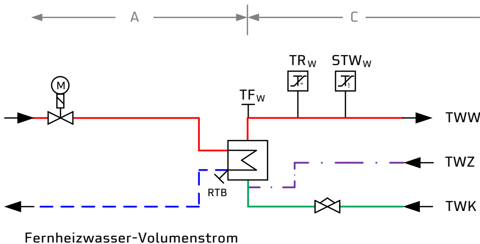
Abbildung 19: Hauszentrale-Trinkwassererwärmung Prinzipschaltbild für den indirekten Anschluss
