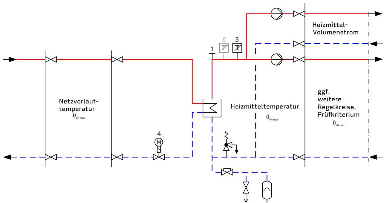
Abbildung 17 zur Tabelle 10: erforderliche sicherheitstechnische Ausrüstung nach Zeile 2; grau dargestellte Komponenten nicht erforderlich
