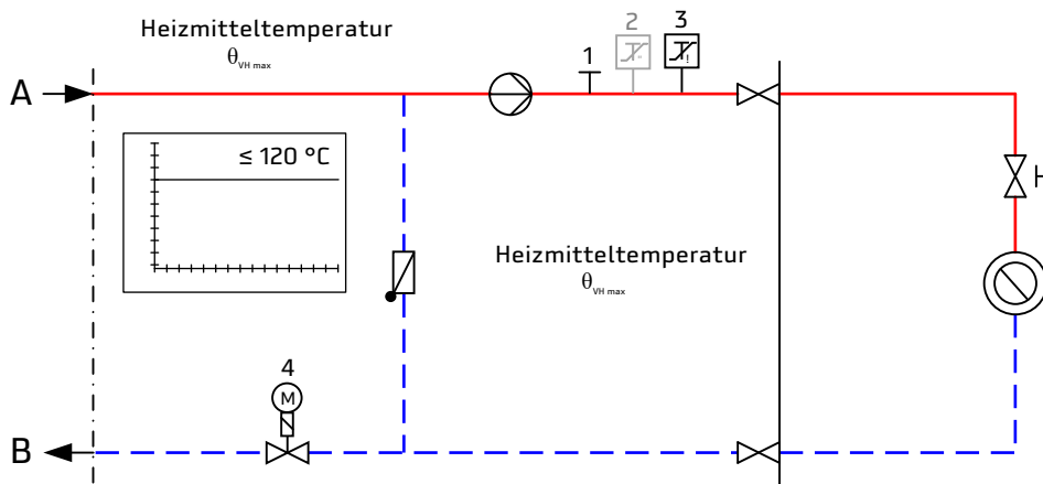
Abbildung 13 zur Tabelle 7: erforderliche sicherheitstechnische Ausrüstung nach Zeile 3; grau dargestellte Komponenten nicht erforderlich
